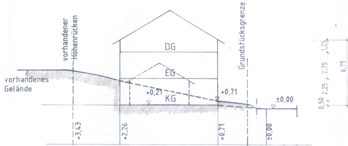
Schnitt 4-1
