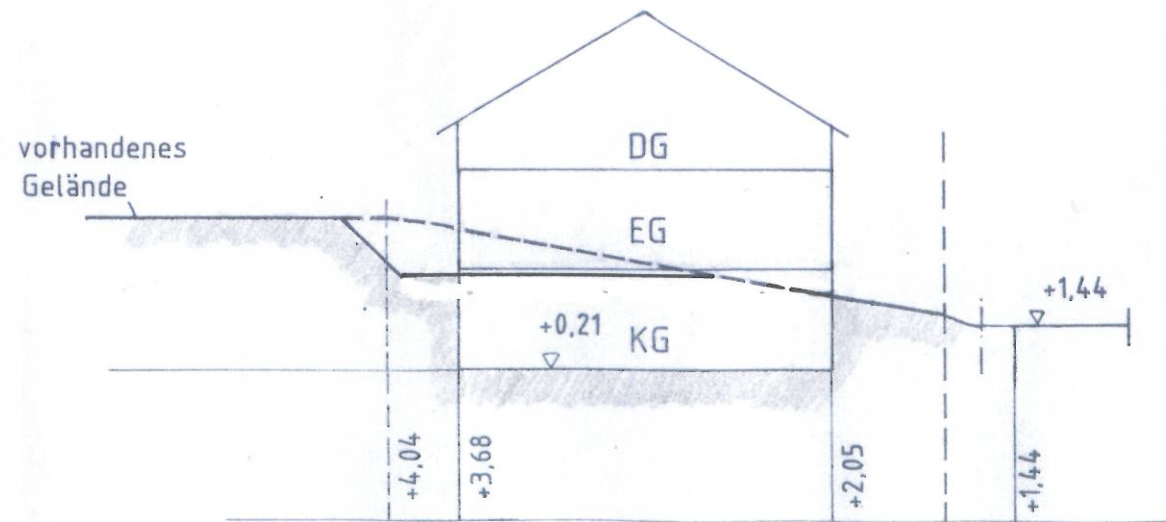
Schnitt 3-2
